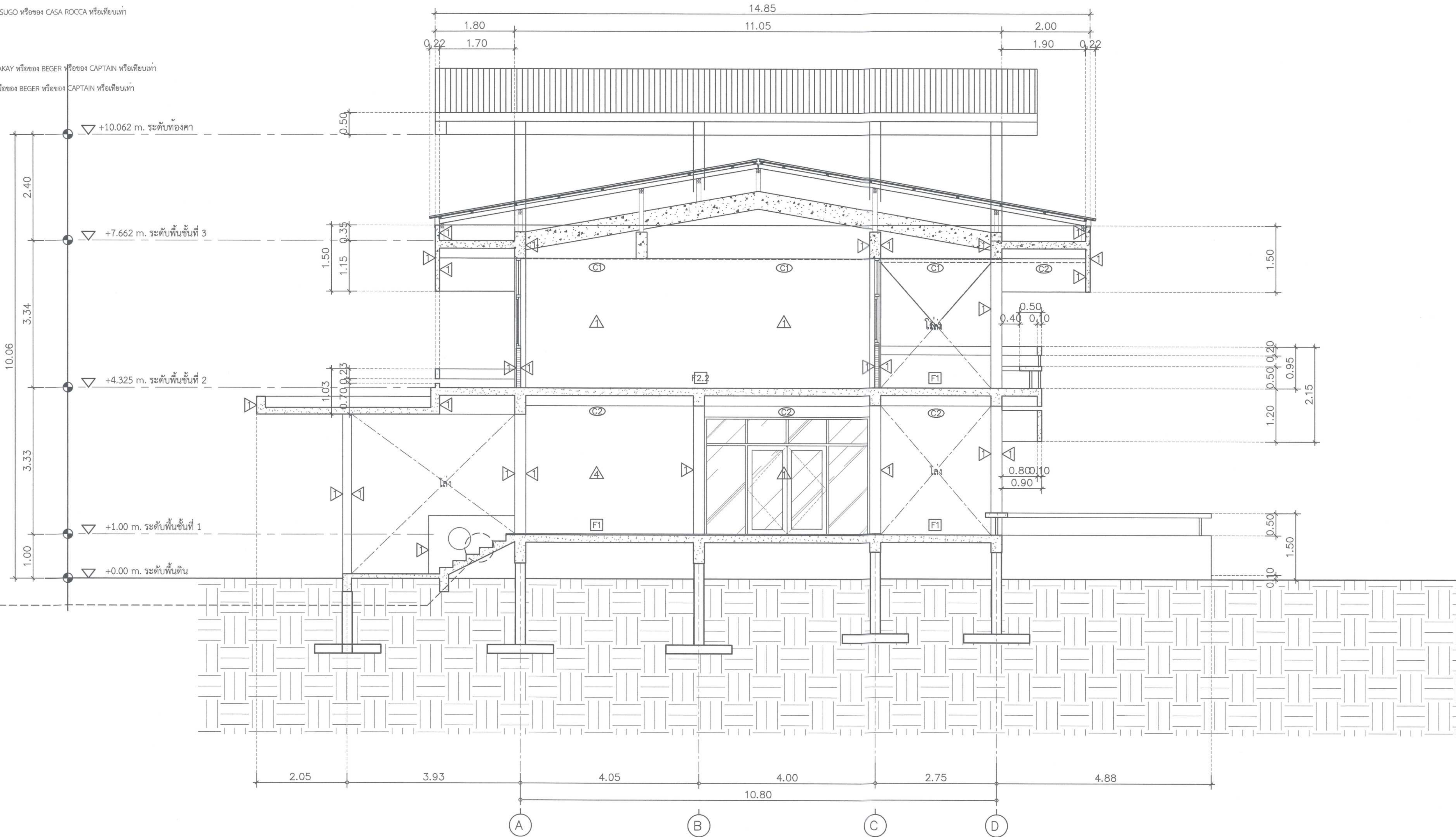
รูปตัด B Scale 1 : 50
